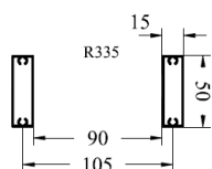
Detalhe perfil R335
